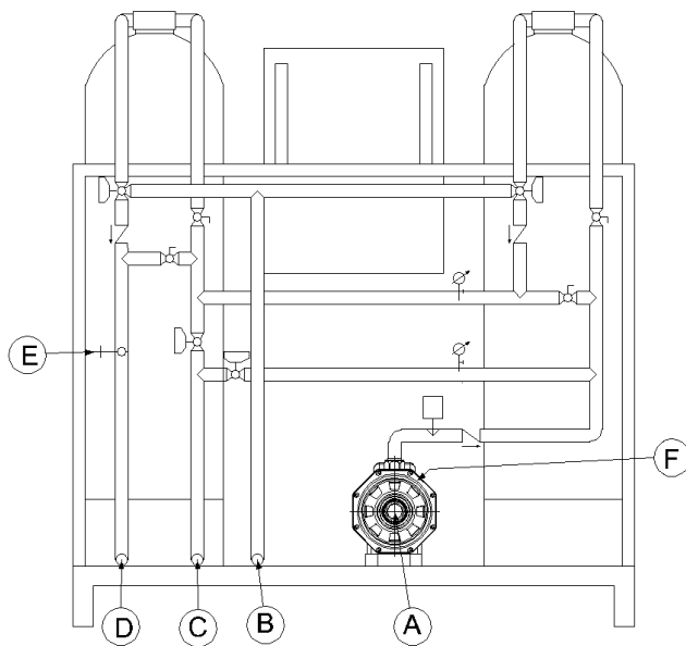
Figura 1 Posizione allacci/collegamenti
