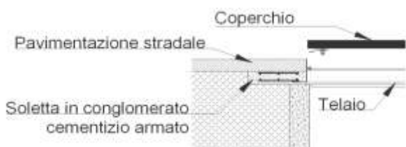
Figura 3 Installazione chiusino quadrangolare
