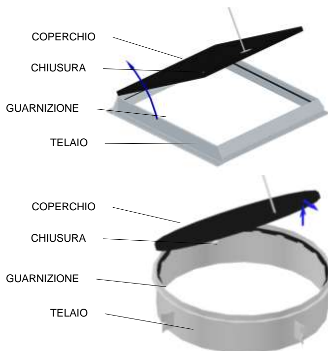
Figura 1 Componenti chiusino circolare e quadrangolare
