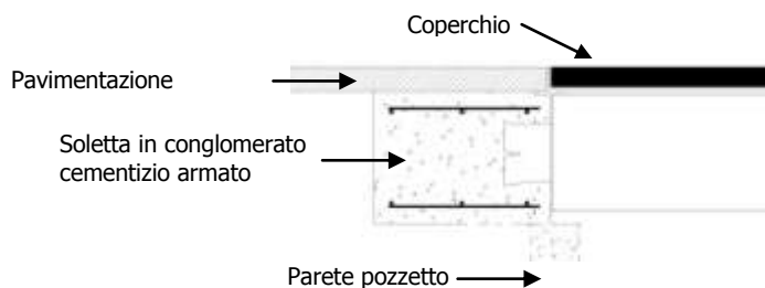
Figura 3 Installazione chiusino quadrangolare
