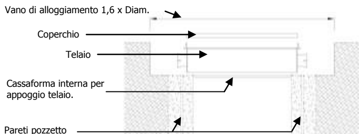
Figura 2 Installazione chiusino circolare
