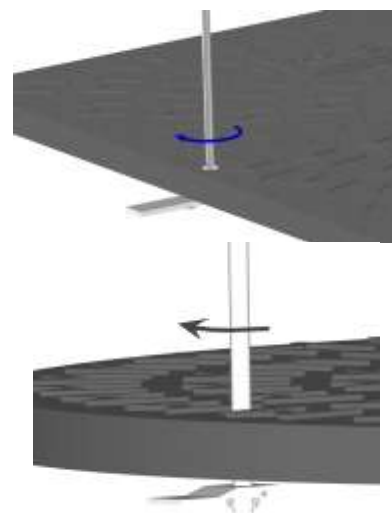
Figura 4 Bloccaggio chiusino circolare e quadrangolare
